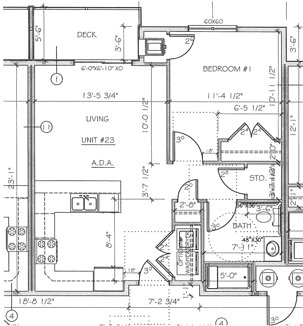
1 A.D.A. UNIT #23 SCALE: 3/16" = 1'-0"
