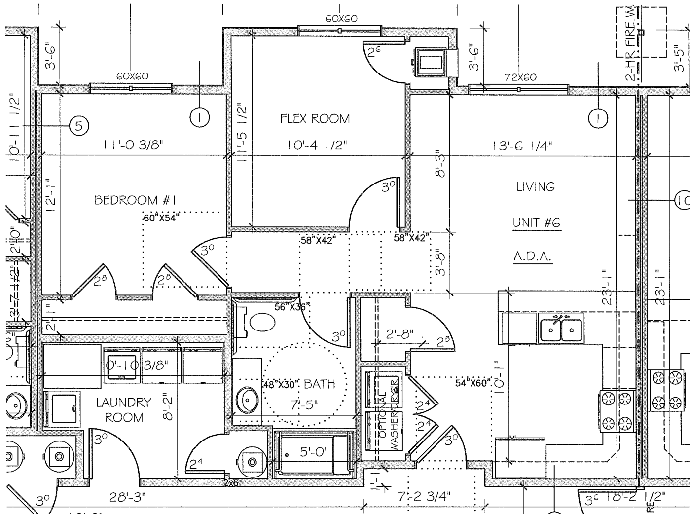
1 A.D.A. UNIT #6 SCALE: 3/16" = 1'-0"
